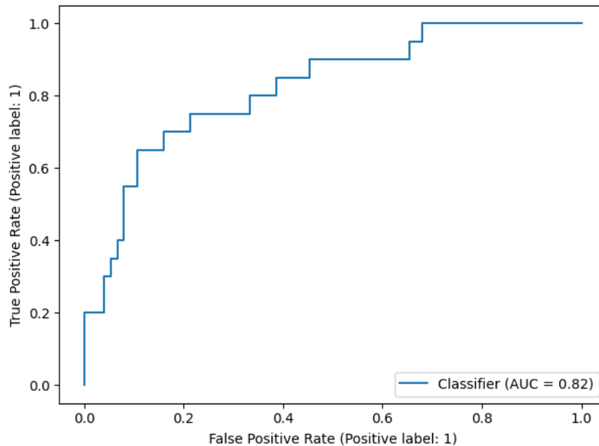
Fig 2. ROC
